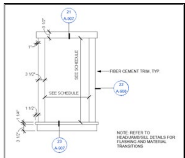
Detalles de la moldería de ventana
