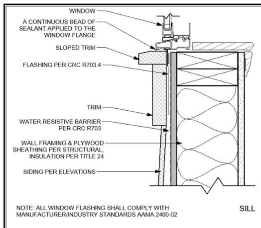
Detalles del alféizar de la ventana
