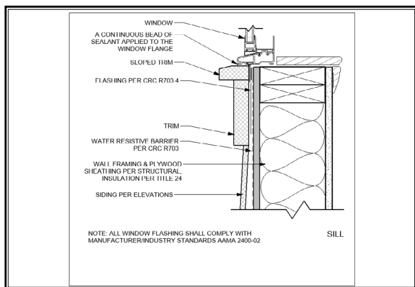
Detalles del alfeizar de la ventana
