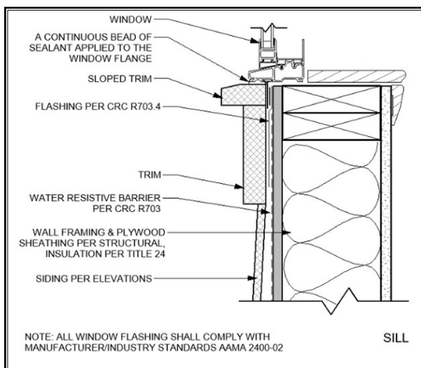
Detalles del alfeizar de la ventana
