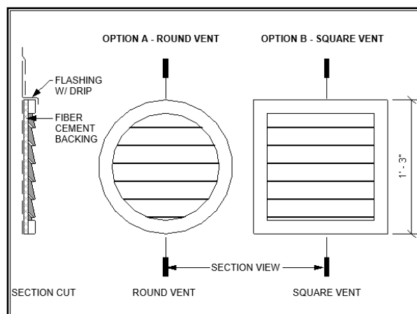
Detalle de ventilación
