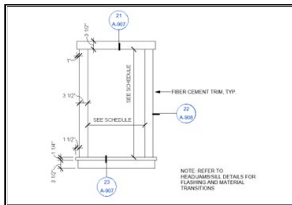
Detalles de la moldería de ventana
